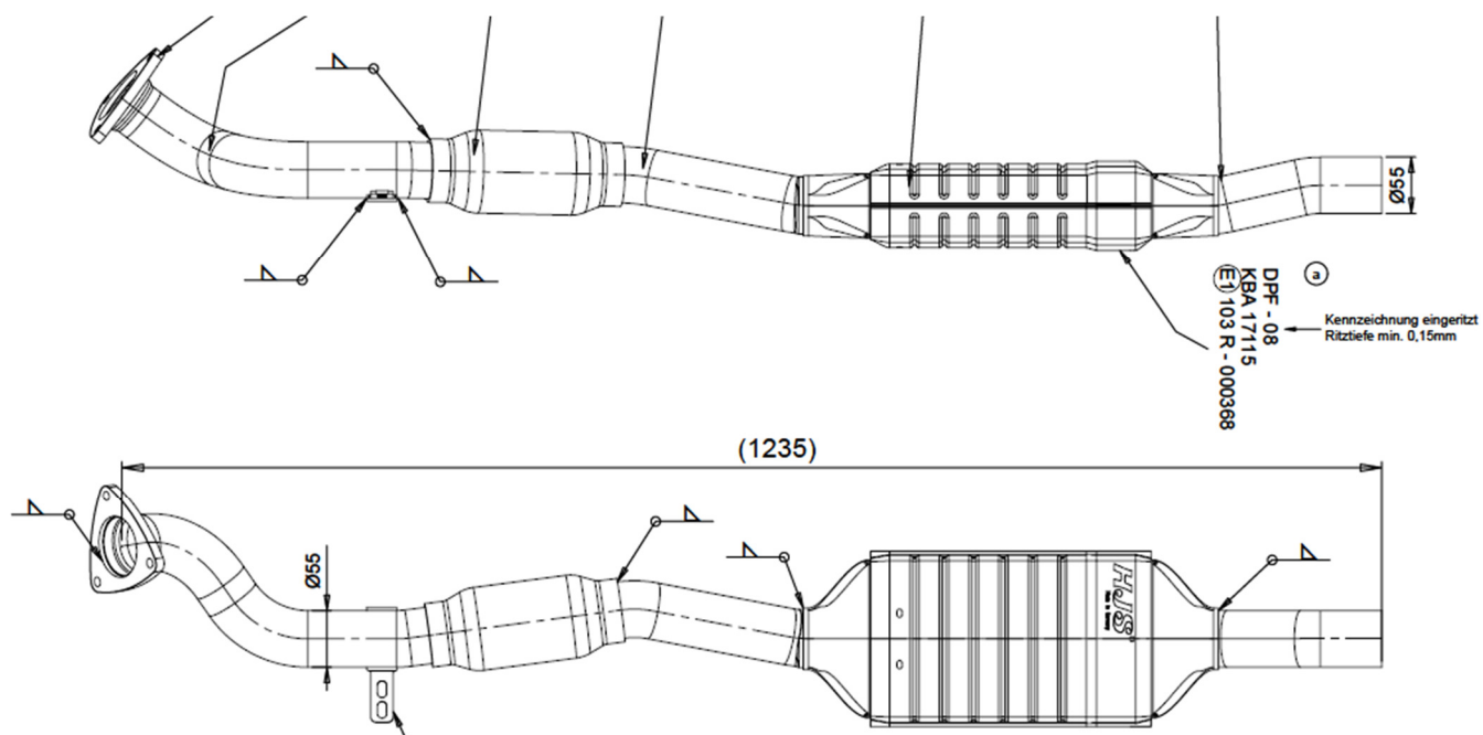
Oprindelig løsning fra HJS, forrør med Partikelfilter.
